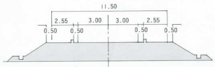
長竿バイパス標準横断面図
